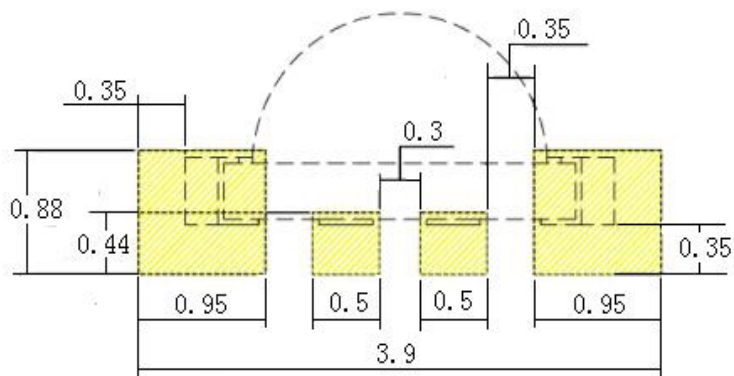
建议焊盘尺寸
