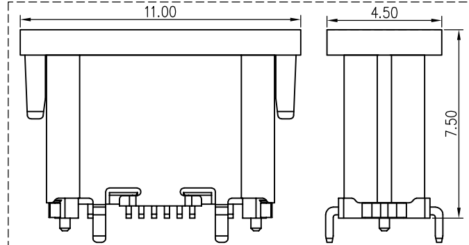
装吸取盖示意图
