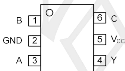
SOT23-6 / SOT363
