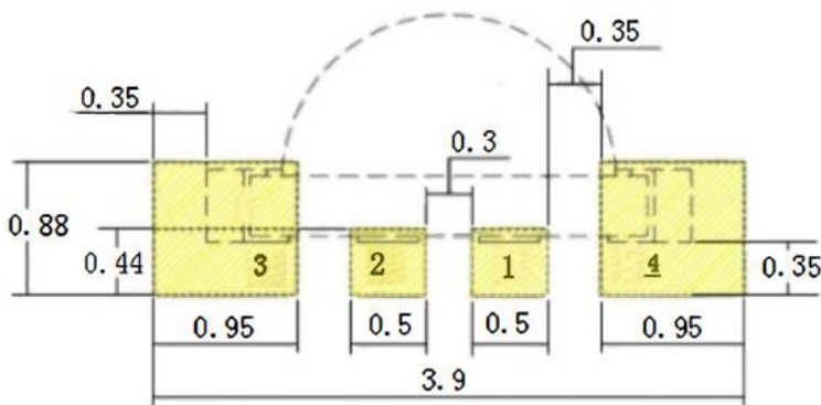
建议焊盘尺寸
