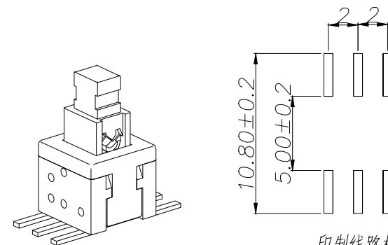
印制线路板 PCB Layout Recommended
