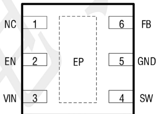
DFN-6(2X2)
