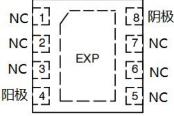
图 5 DFN-8 管脚图
