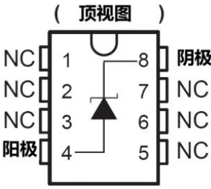
图 4 SOP8/MSOP8 管脚图
