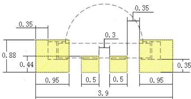
建议焊盘尺寸
