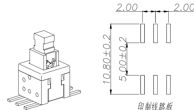
印制线路板 PCB Layout Recommended
