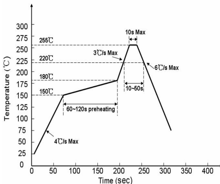
无铅制程
