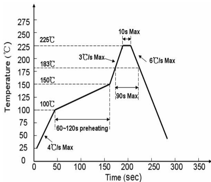
有铅制程
