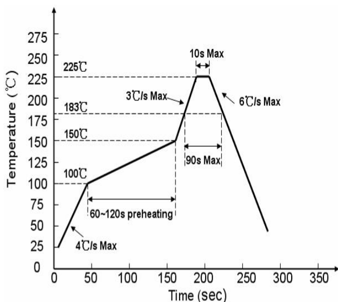
有铅制程
