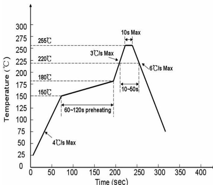
无铅制程
