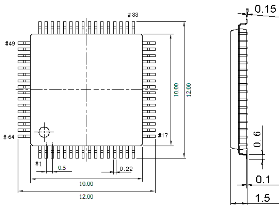
图 5-4 LQFP64M 封装
