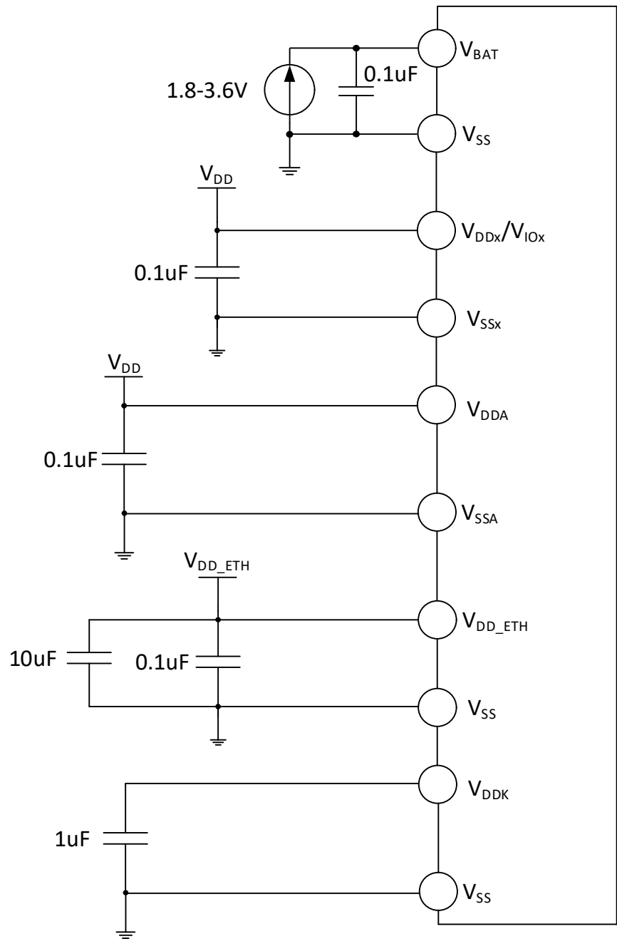
图 4-1-2 CH32V317 常规供电典型电路
