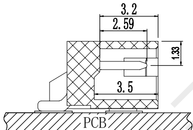
剖面 A-A
