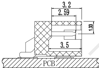
剖面 A-A
