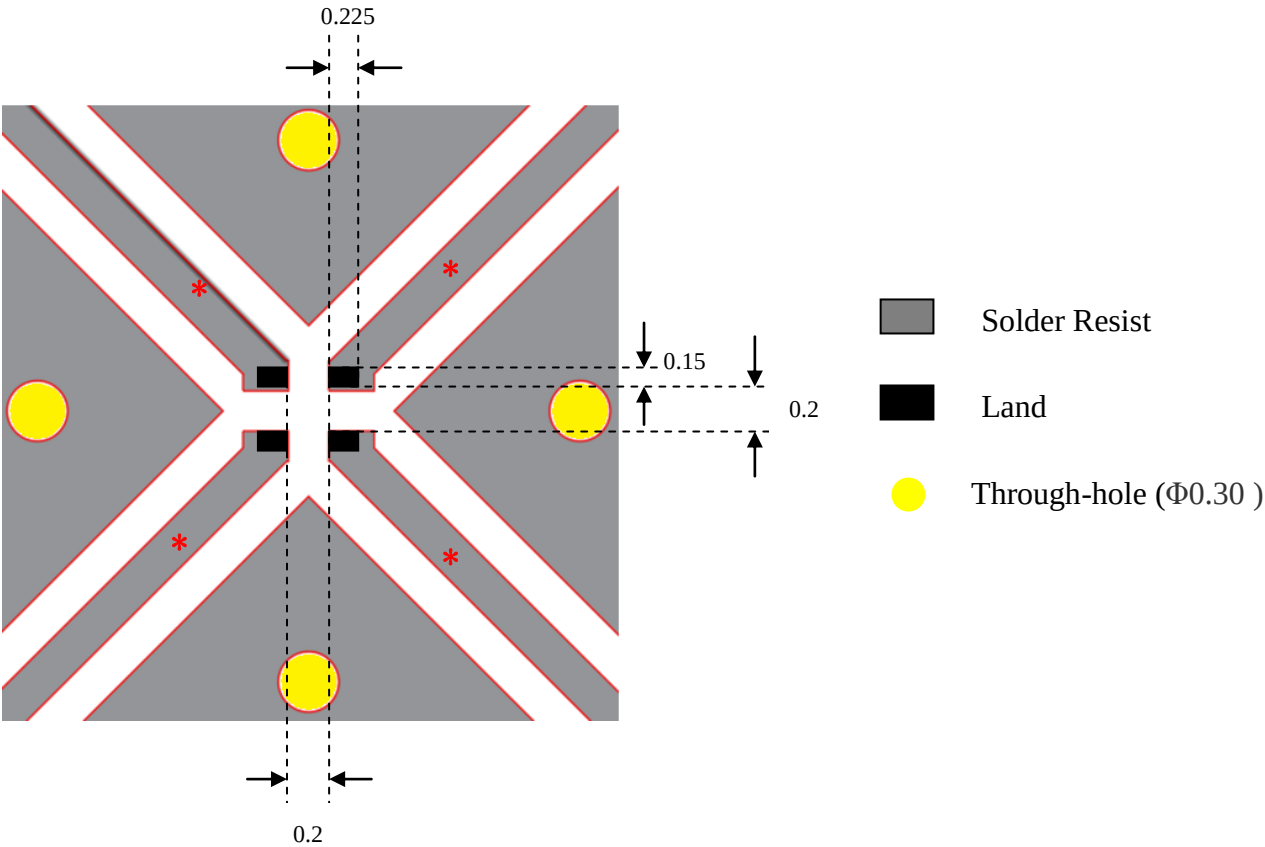
建议的 PCB 布局 ( Recommended PCB Layout )
