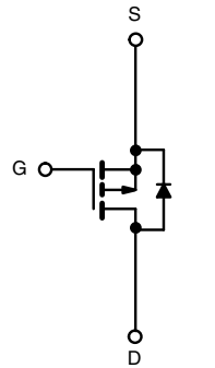
P-Channel MOSFET
