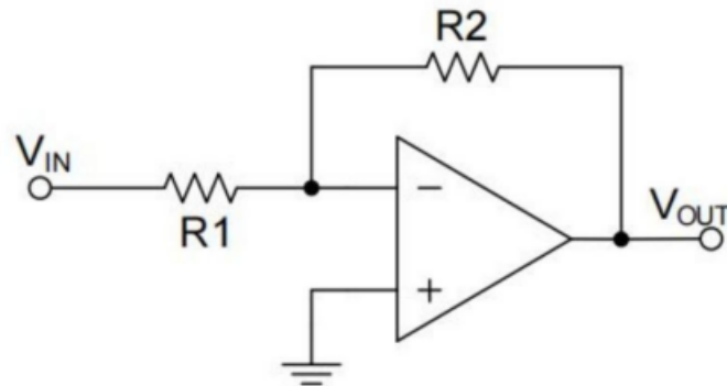
图1 反向放大器
