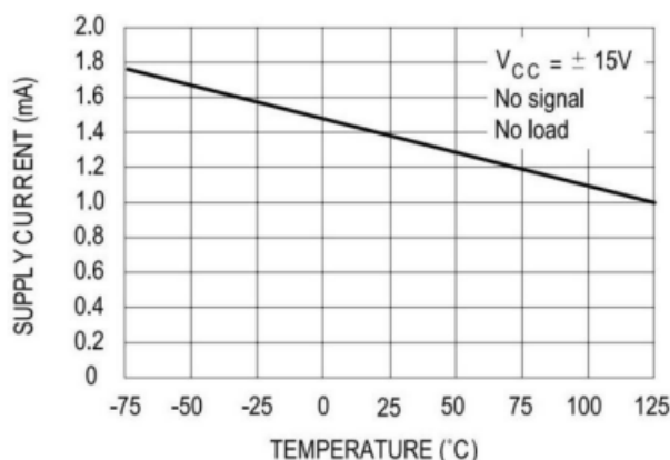
图4 电源电流与环境温度关系 (每通道)
