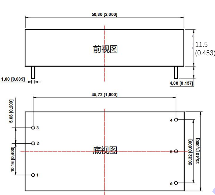
URB_LD-60WR3系列外观尺寸图
