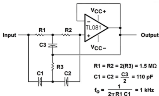
图2 高品质陷波滤波器
