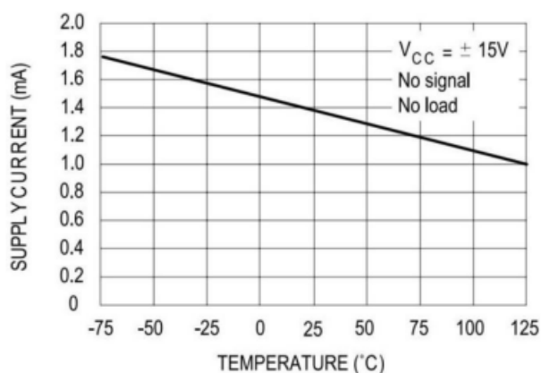
图4 电源电流与环境温度关系
