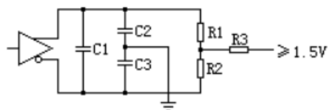
图9-3 3态(低)测试负载电路图和波形图
