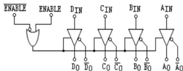
图4-1 26C31功能模块框图
