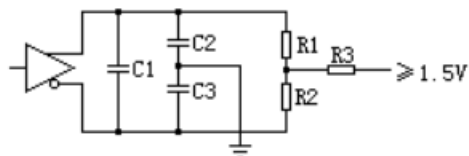
图9-4 3态(高)测试负载电路图和波形图
