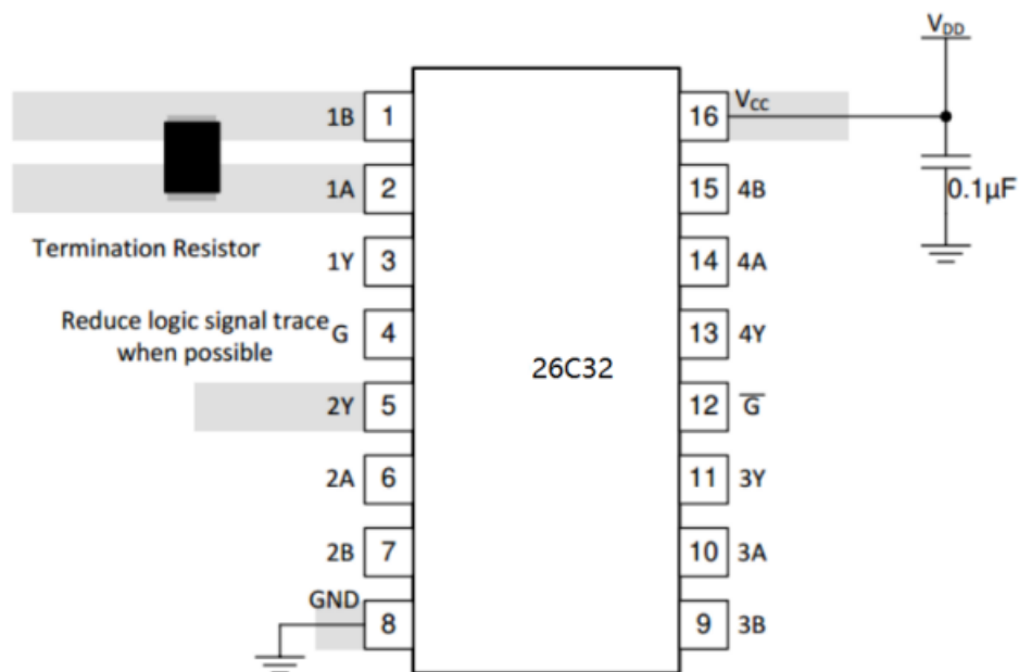
图10-2 实例电路
