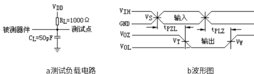
图9-2 3态(低)测试负载电路a和波形图b
