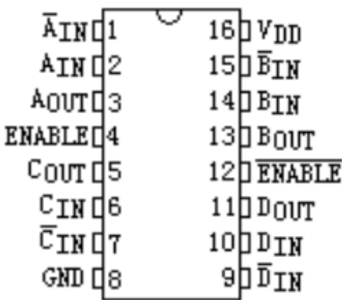
图7-1 引出端排列
