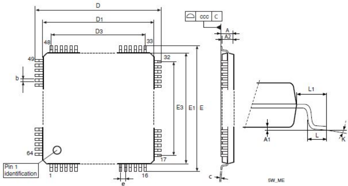
图 26 LQFP64-10x10mm, 64 脚低剖面方形扁平封装图
