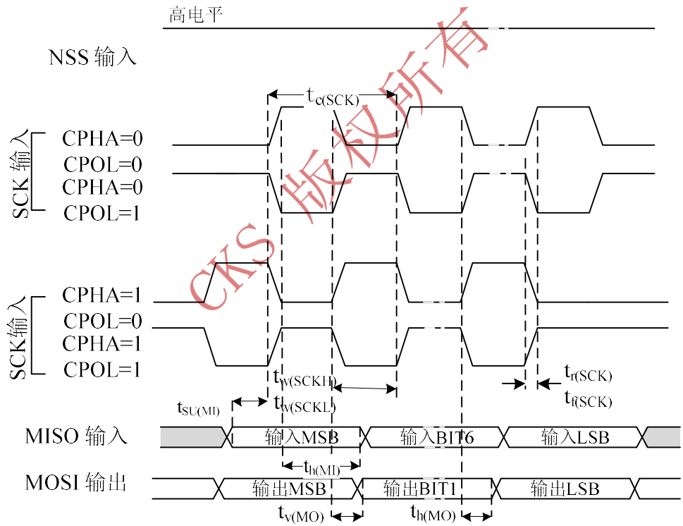
图 28 SPI 时序图-主模式 (1)
