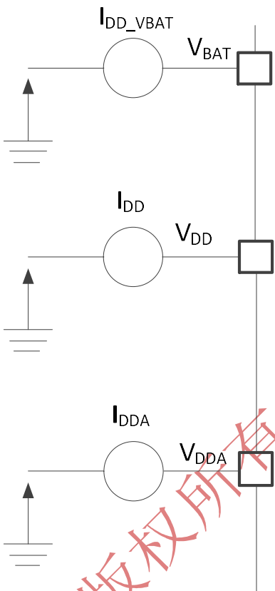
图 12 电流消耗测量方案
