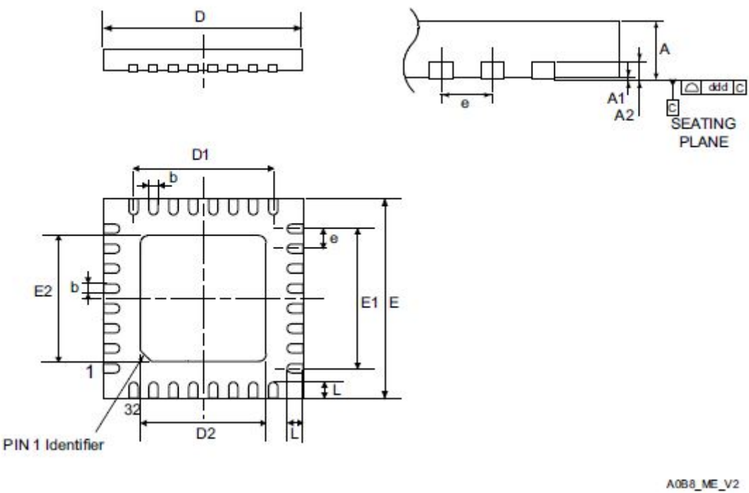
图 39 UFQFPN32 封装外形 (1)
