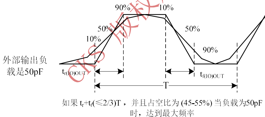
图 21 输入输出交流特性定义
