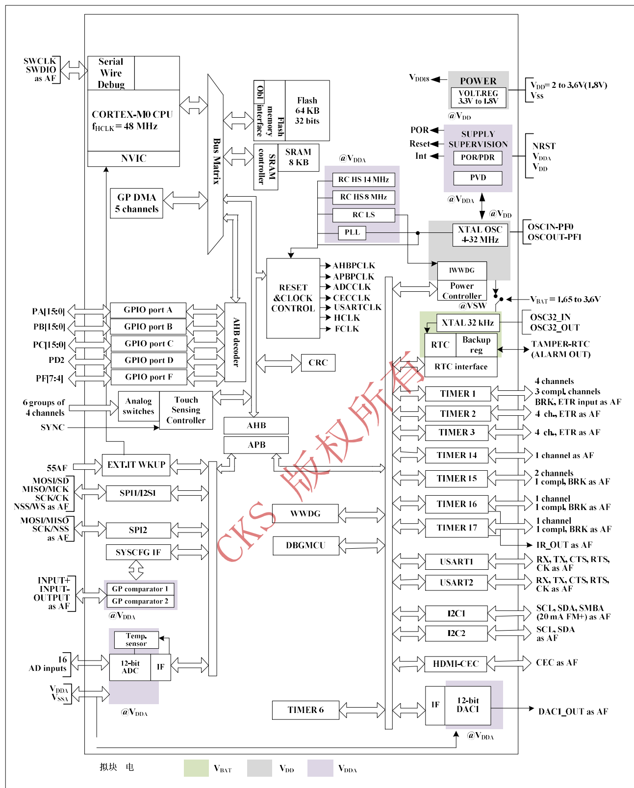
图 1 模块图
