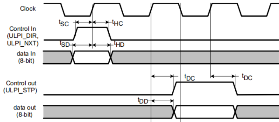
图 24 ULPI 时序图
