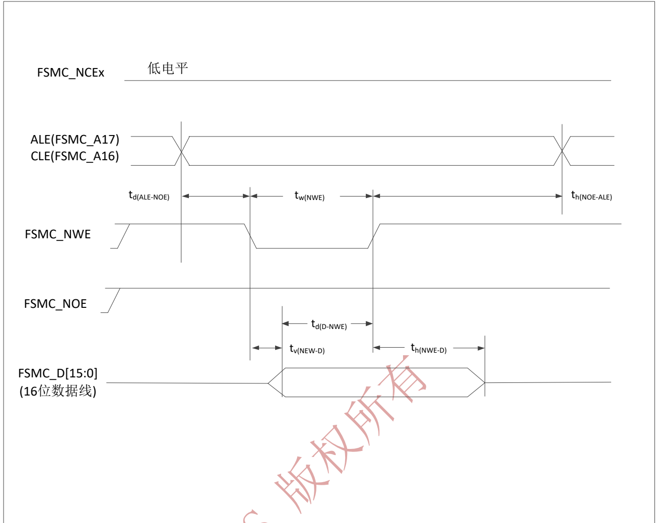
图 50 NAND 控制器在通用存储空间的写操作波形
