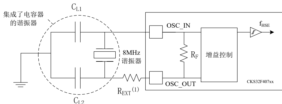
图 14 使用 8MHz 晶体的典型应用
