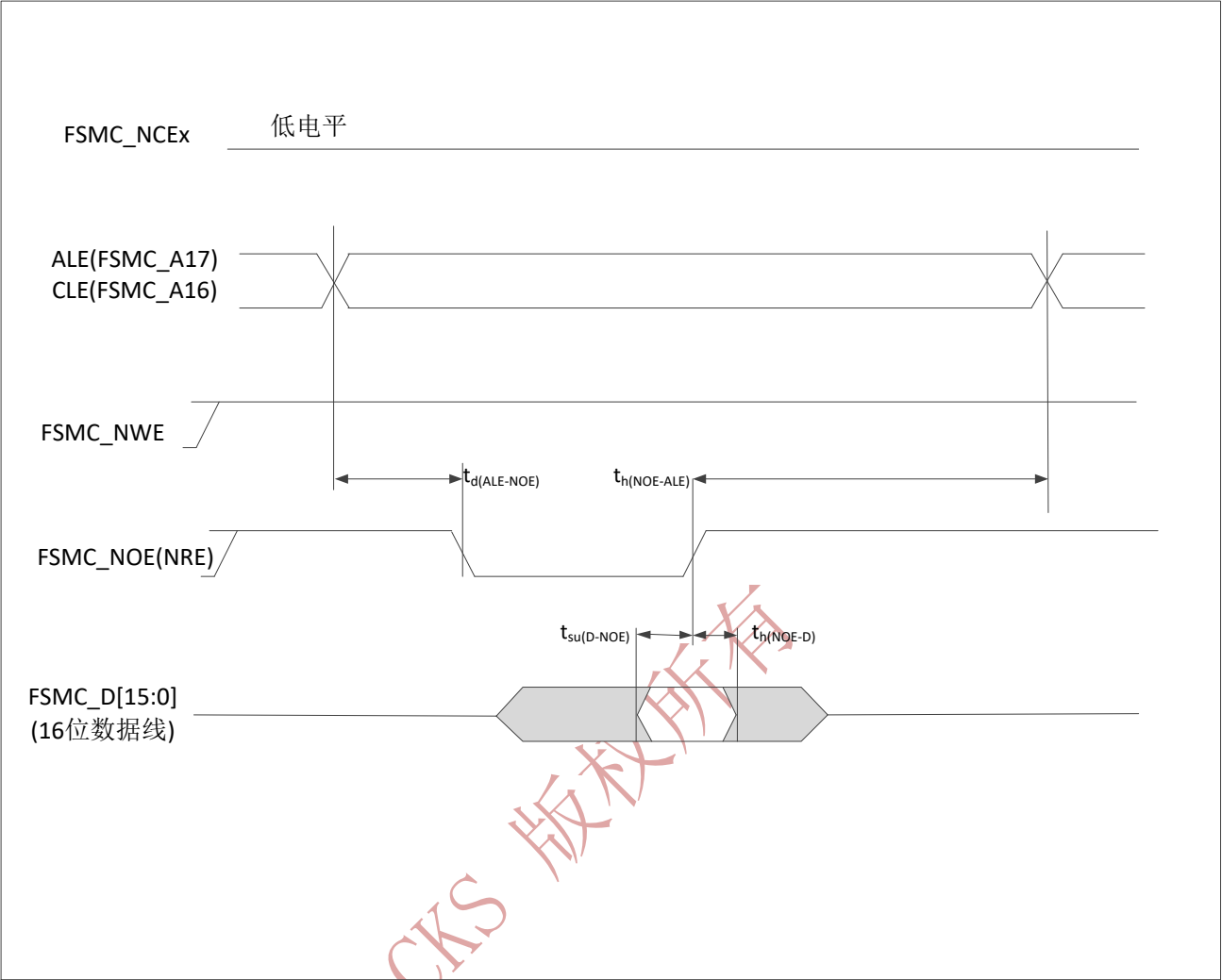
图 47 NAND 控制器读操作波形
