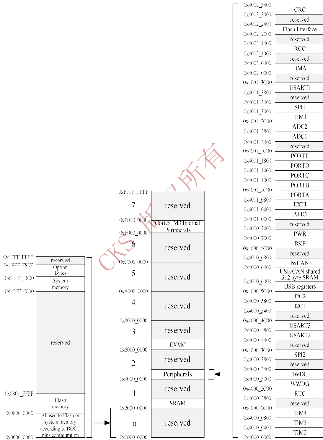
图 8 存储器 MAP 图
