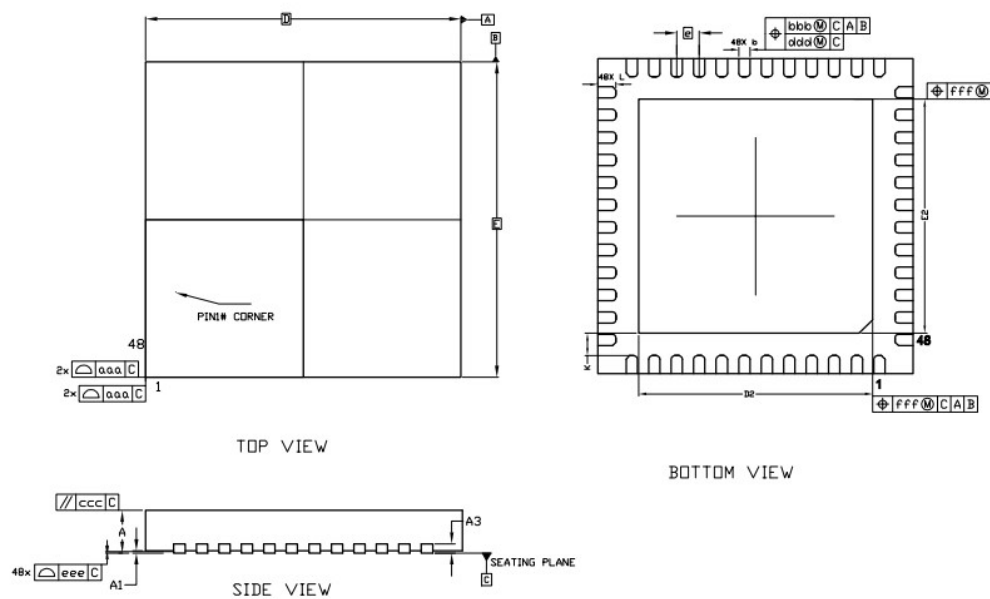
图 29 QFN48 封装图
