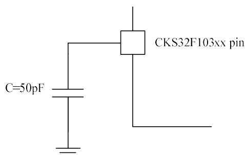
图 9 引脚的负载条件
