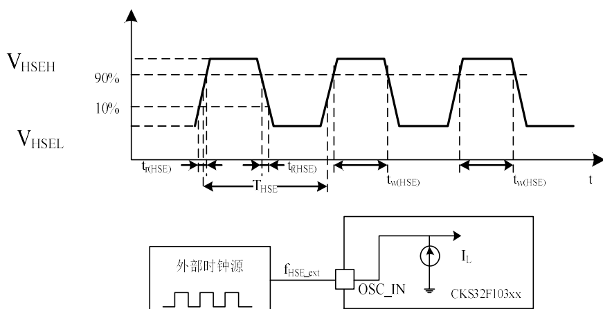
图 13 外部高速时钟源的交流时序图
