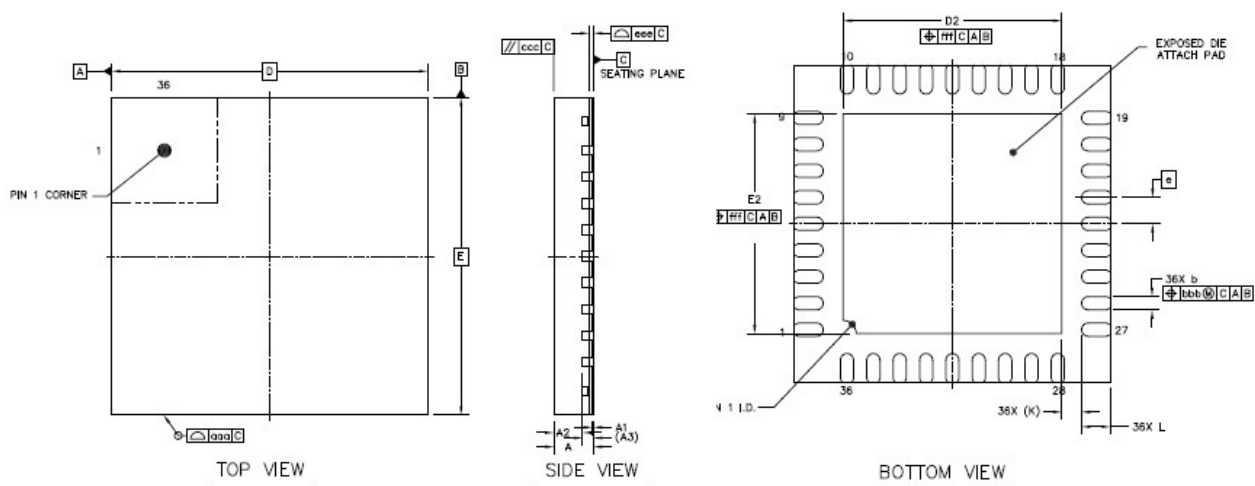
图 28 QFN36 封装图
