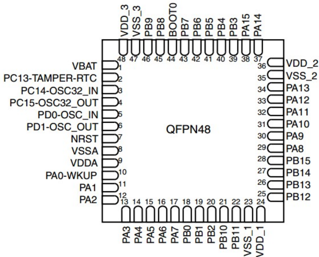
图 6 CKS32F103xx 标准型 QFPN48 引脚分布
