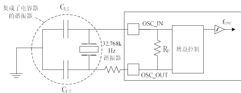
图 16 使用 32.768kHz 晶体的典型应用
