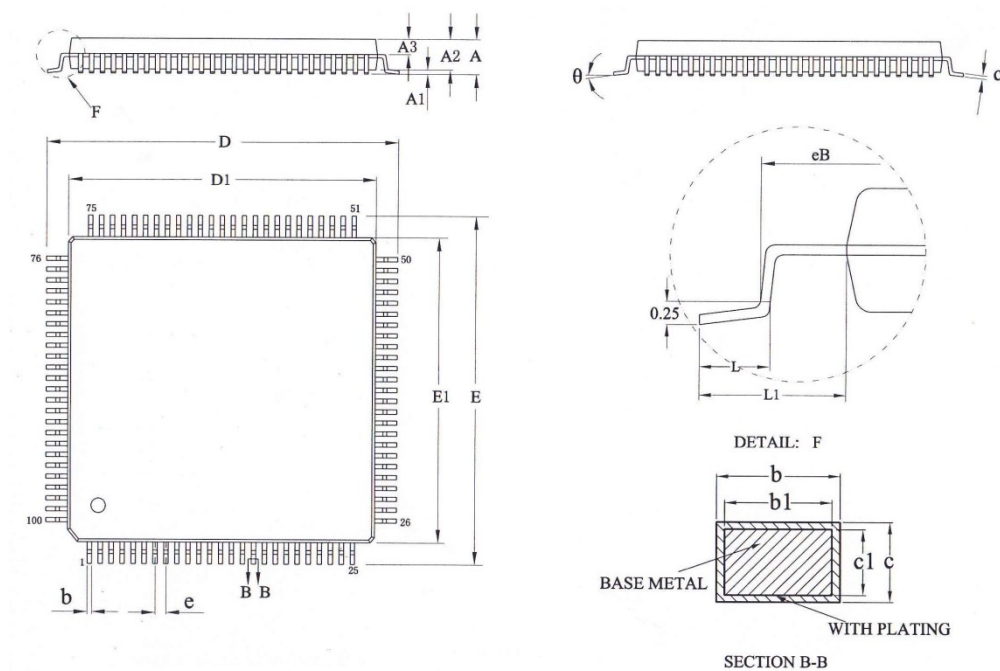
图 30 LQFP100, 100 脚低剖面方形扁平封装图
