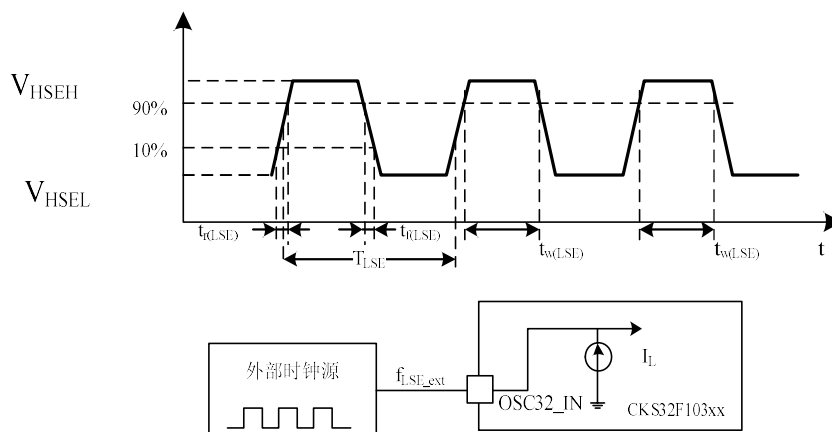
图 14 外部低速时钟源的交流时序图
