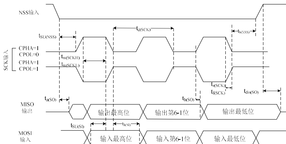
图 21 SPI 时序图- 从模式和 CPHA=1 (1)
