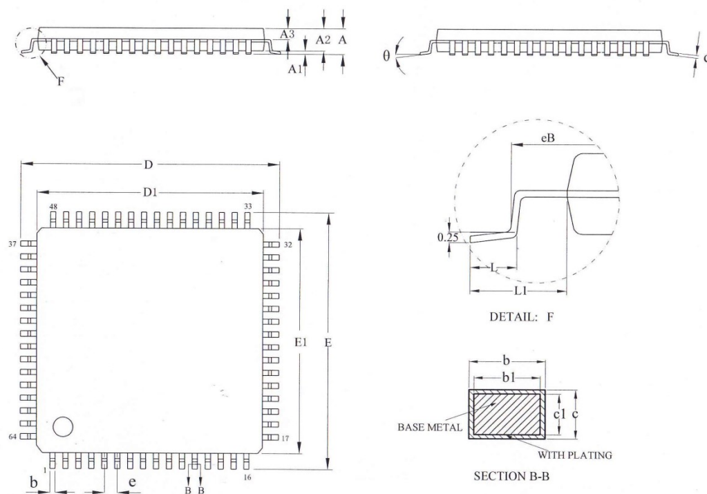
图 31 LQFP64, 64 脚低剖面方形扁平封装图
