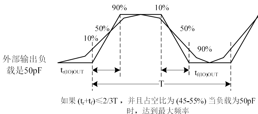
图 17 输入输出交流特性定义
