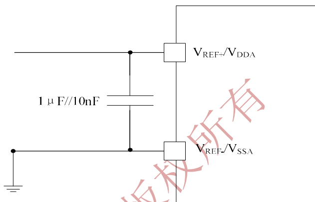
图 27 供电电源和参考电源去藕线路( V_{REF+} 与 V_{DDA} 相连)
