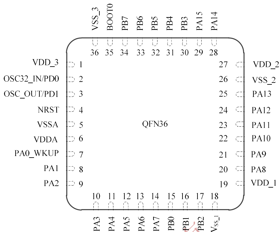
图 7 CKS32F103xx 标准型 QFN36 引脚分布
