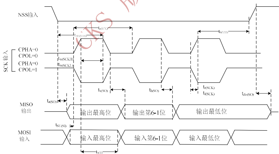
图 20 SPI 时序图-从模式和 CPHA=0
