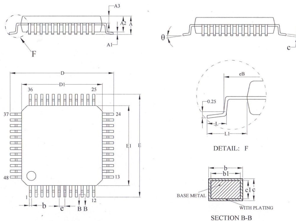
图 32 LQFP48，48 脚低剖面方形扁平封装图
