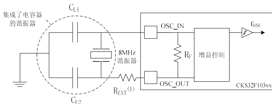
图 15 使用 8MHz 晶体的典型应用
