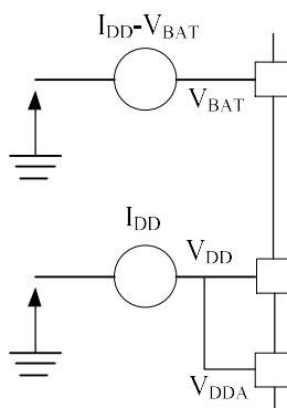
图 12 电流消耗测量方案
