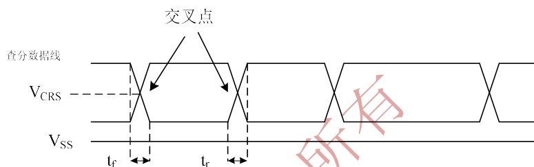
图 23 USB 时序：数据信号上升和下降时间定义
