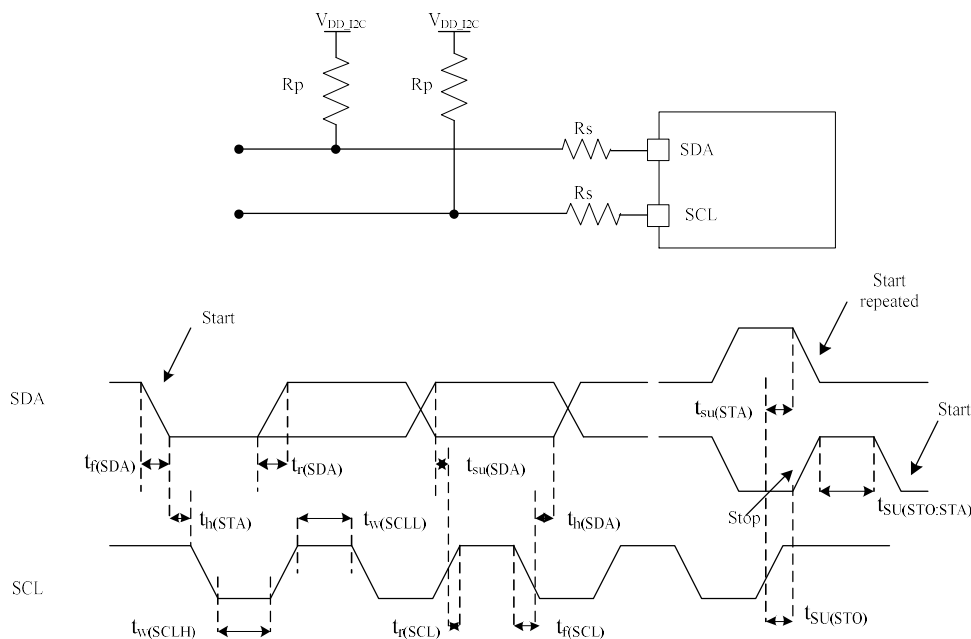
图 19 I 2 C 总线交流波形和测量电路 (1)
