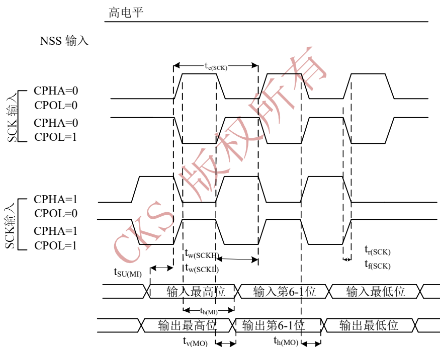
图 22 SPI 时序图-主模式 (1)
