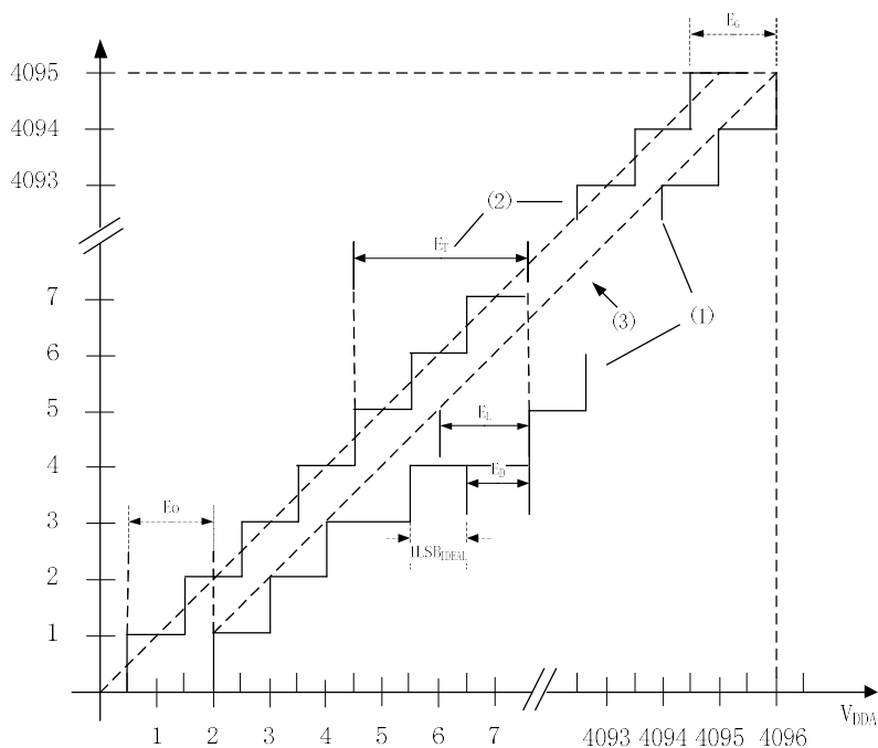
图 24 ADC 精度特性
