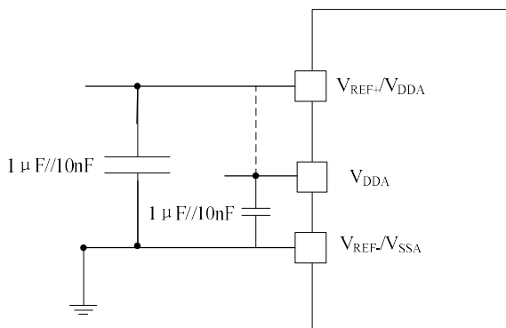
图 26 供电电源和参考电源去藕线路( V_{REF+} 未与 V_{DDA} 相连)
