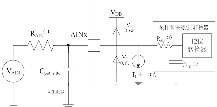
图 25 使用 ADC 典型的连接图
