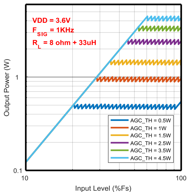
OUTPUT POWER VS. Din
