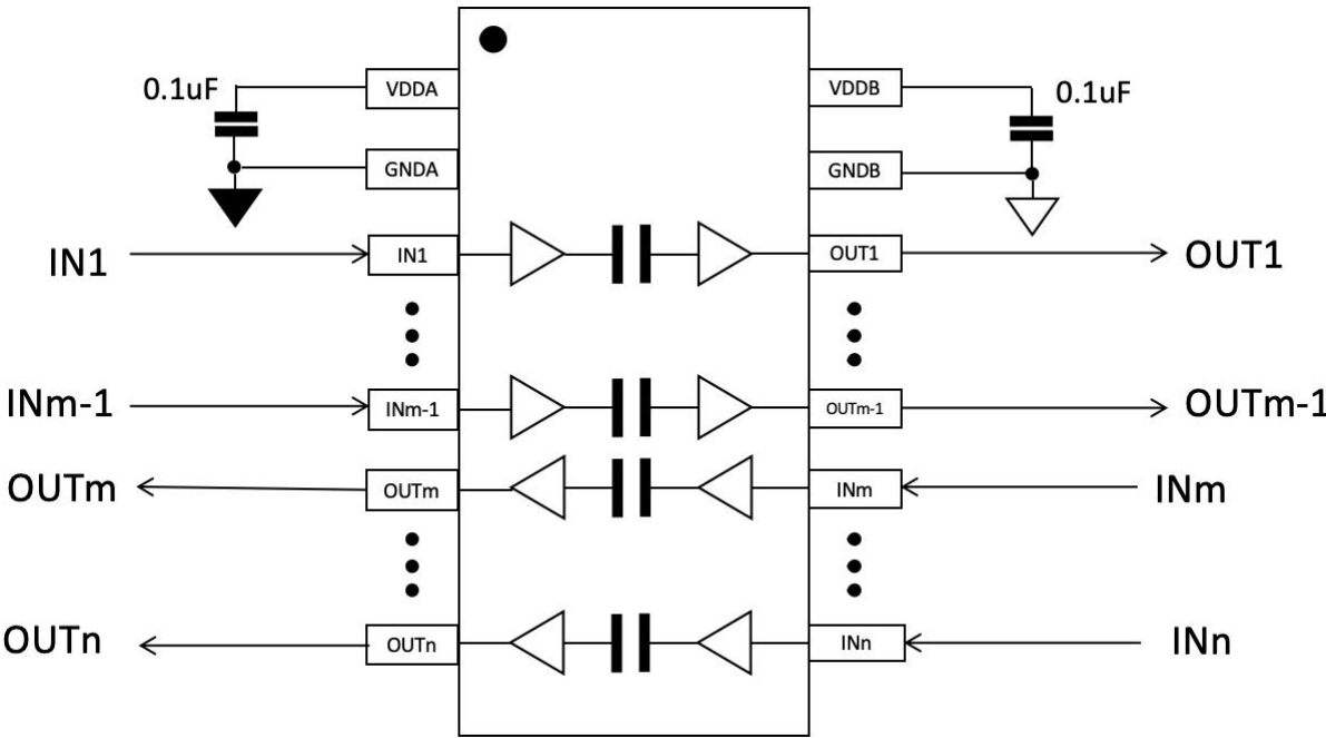
图 6-1 SOW-16 SI862x 典型应用电路
