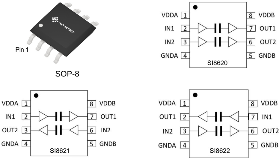
图 2-1 SI862x SOP-8 封装顶部视图
