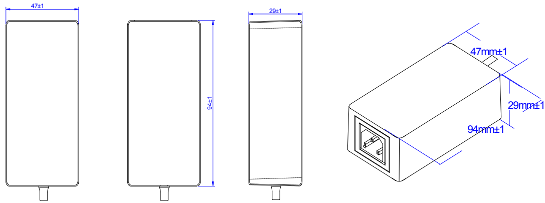
品字尾 IEC320-C14
