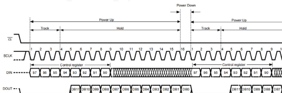
XADC122S021 操作时序图
