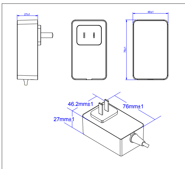
中规插脚
