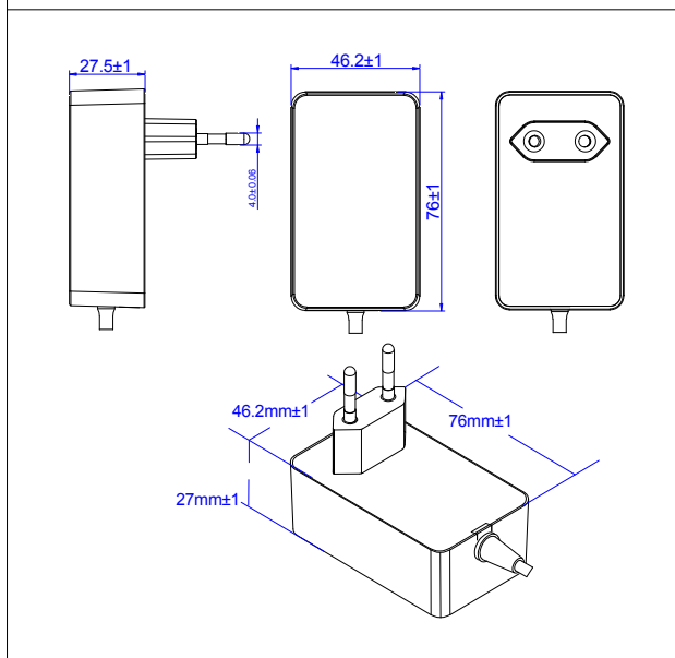
欧规插脚
