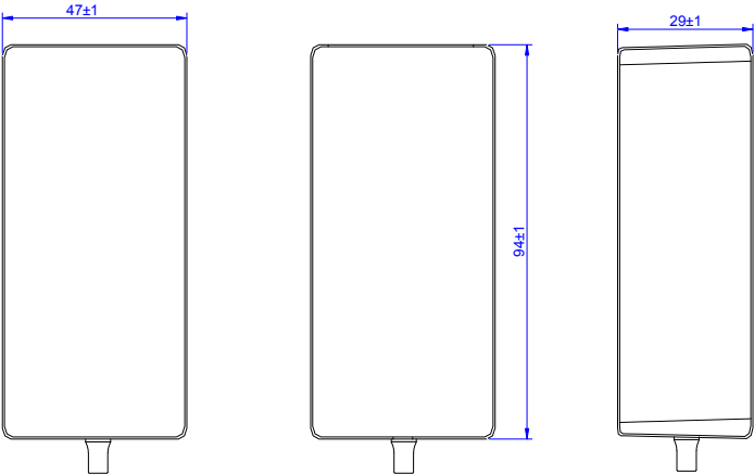
梅花尾 IEC320-C6
