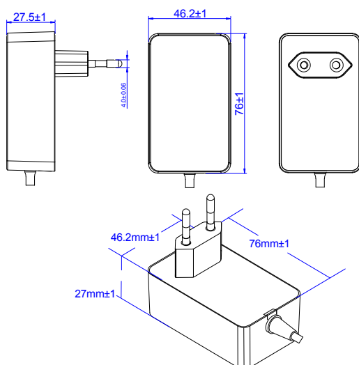
欧规插脚
