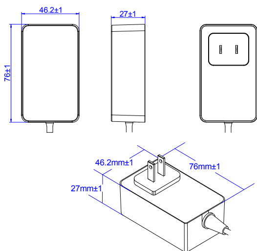
美规插脚
