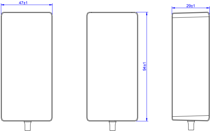
品字尾 IEC320-C14
