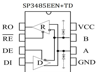
图 1 SP3485EEN+TD引脚分布图
