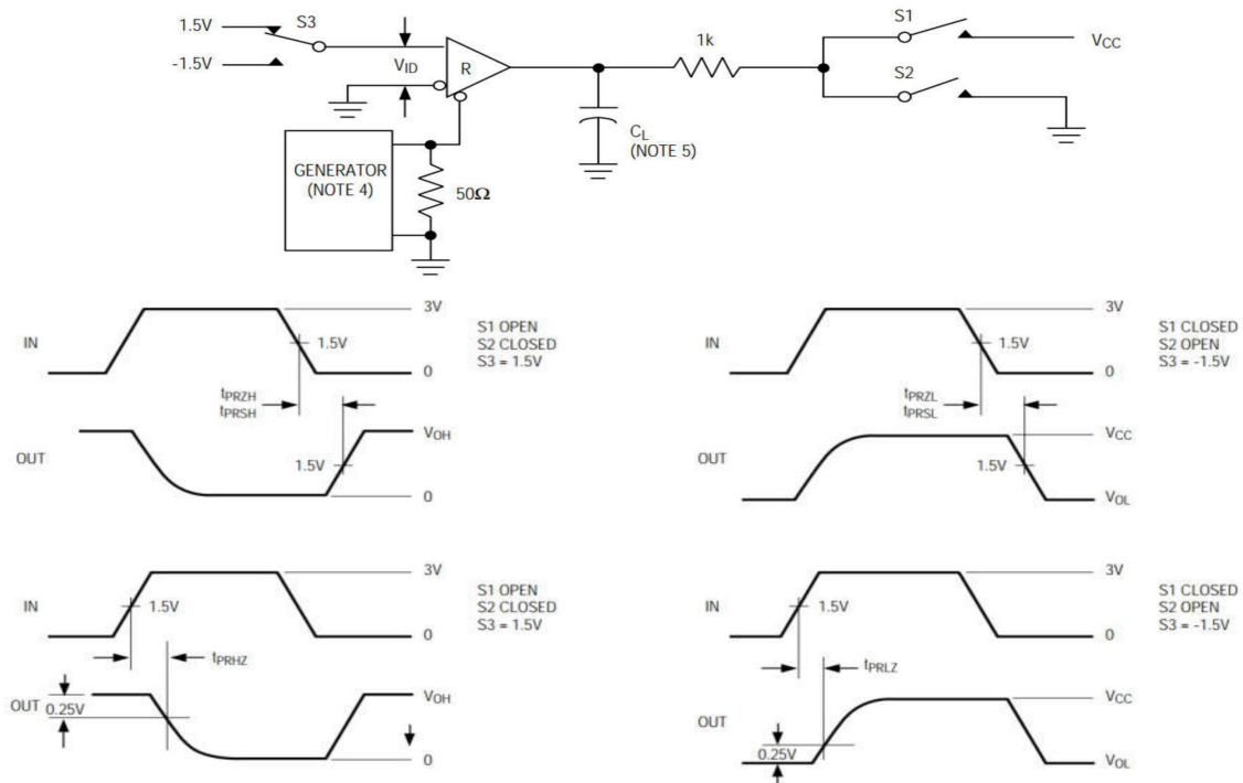
图 8 接收器使能与禁能时间
