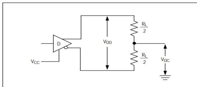
图 2 驱动器直流测试负载
