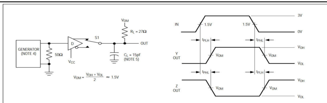
图 4 驱动器传播延迟
