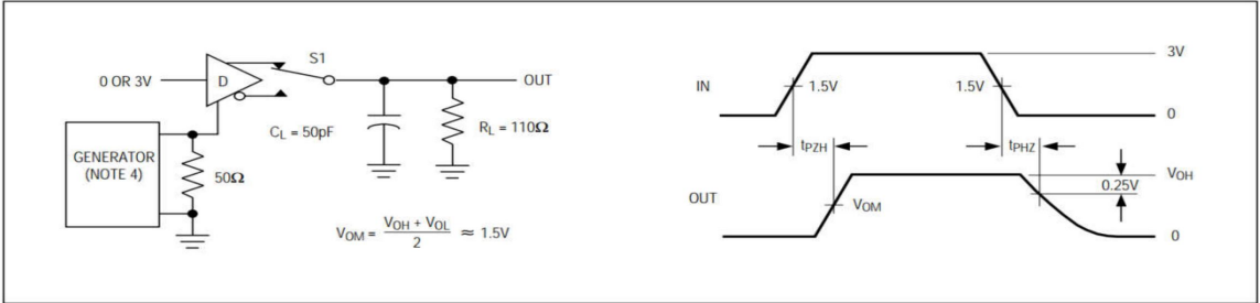
图 5 驱动器使能与禁能时间
