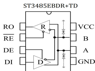
图 1 ST3485EBDR+TD 引脚分布图
