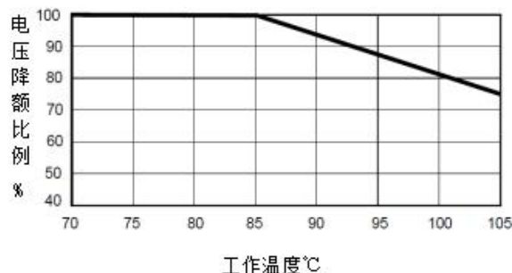
额定电压降额曲线
