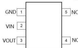
SOT23-5B
