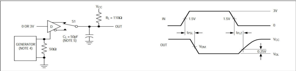
图 6 驱动器使能与禁能时间
