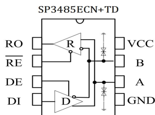
图 1 SP3485ECN+TD引脚分布图
