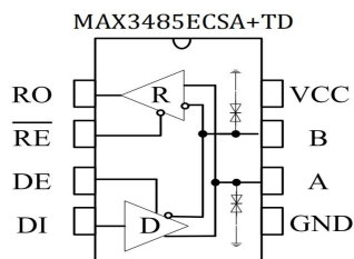
图 1 MAX3485ECSA+TD 引脚分布图
