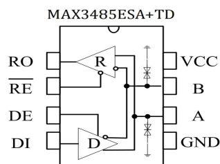
图 1 MAX3485ESA+TD引脚分布图
