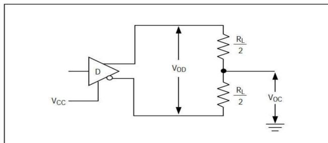
图 2 驱动器直流测试负载
