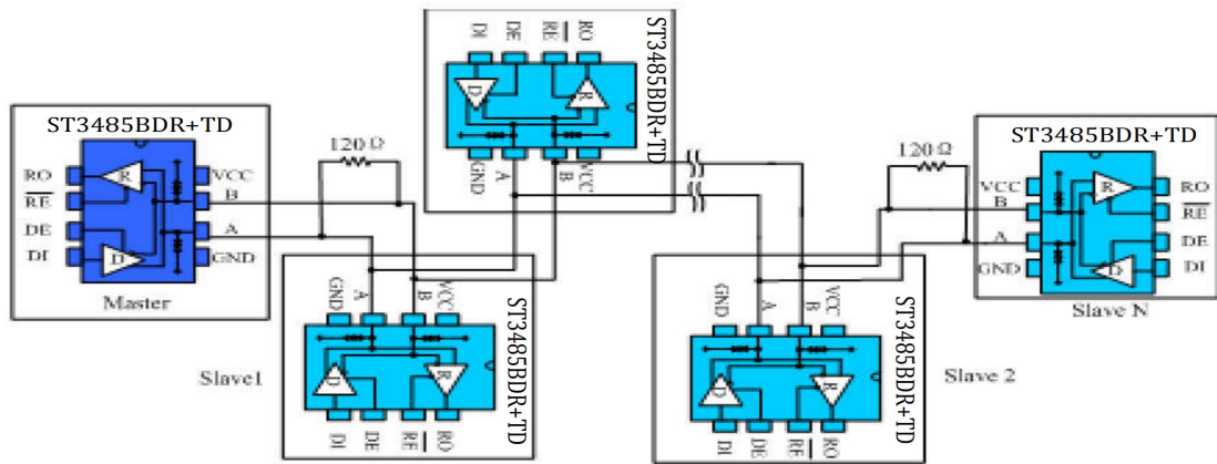
图 10 手拉手式 RS485 半双工通讯网络
