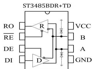
图 1 ST3485BDR+TD引脚分布图
