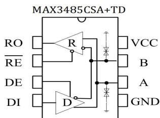
图 1 MAX3485CSA+TD引脚分布图
