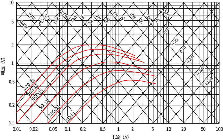
XXD-11电压-电流曲线
