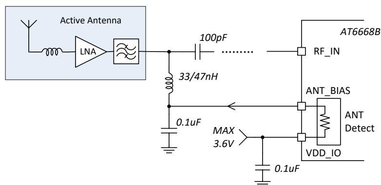
图 5-3 有源天线检测和保护的电路示意图
