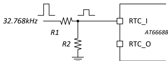
图 5-5 32kHz 直接时钟输入（电阻分压）
