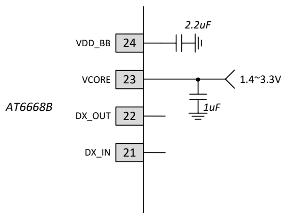
图 5-2 内核 LDO 由外部电源直接供电方案
