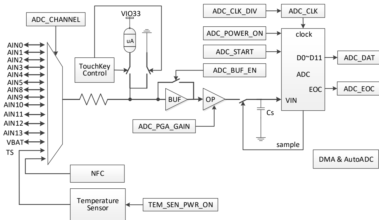
图 15-1 ADC 结构图
