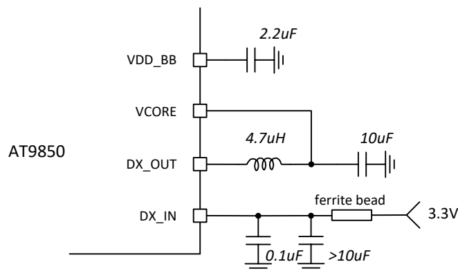
图 5-8 如果电源串联磁珠, 需要较大的滤波电容
