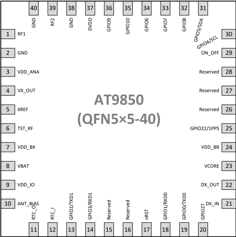
图 2-1 AT9850 芯片封装管脚排列
