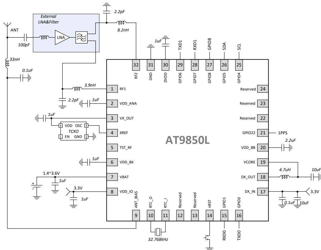
图 5-2 AT9850L 芯片参考设计方案
