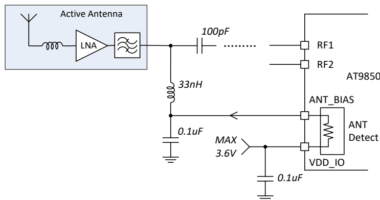
图 5-5 有源天线检测和保护
