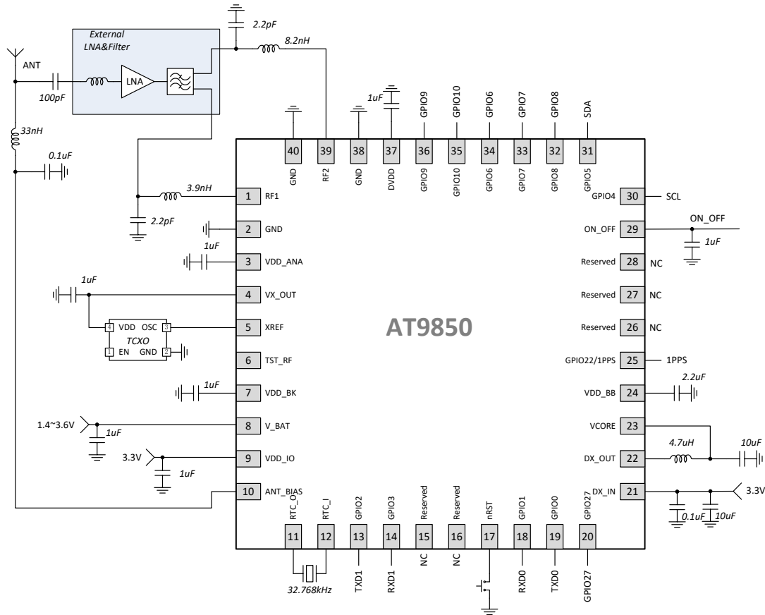
图 5-1 AT9850 芯片参考设计方案
