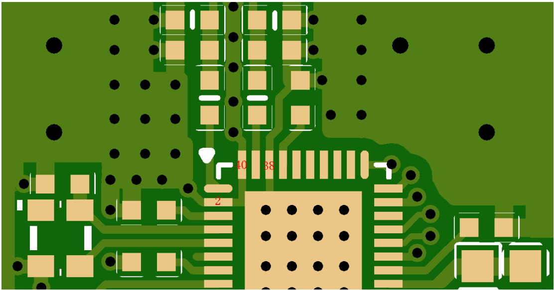
图 5-3 AT9850 射频输入信号隔离
