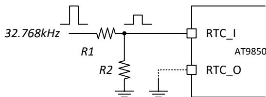
图 5-7 RTC 时钟采用 32.768kHz 直接输入
