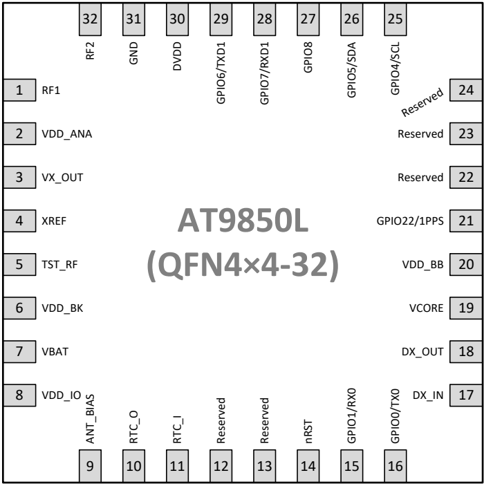
图 2-2 AT9850L 芯片封装管脚排列
