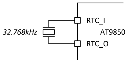
图 5-6 RTC 时钟采用 32.768kHz 无源晶体
