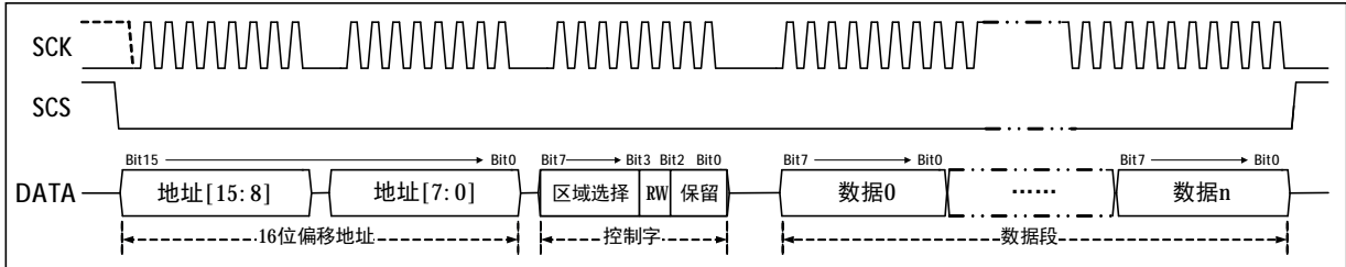
图 5-1 CH394Q 数据帧
