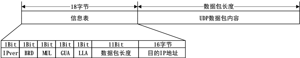
图 12-2 IPRAW6 模式下接收数据包格式
