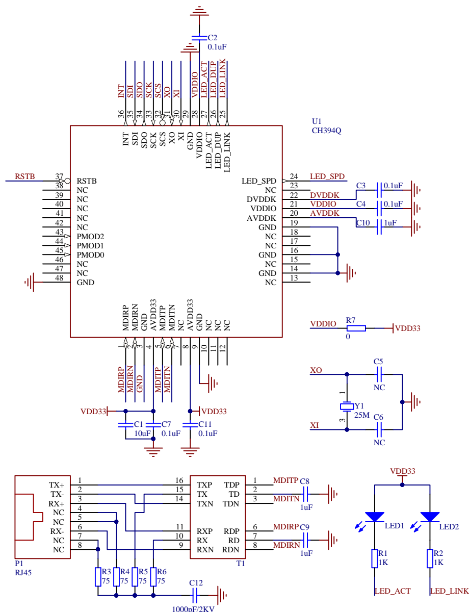
图 12-3 硬件参考电路
