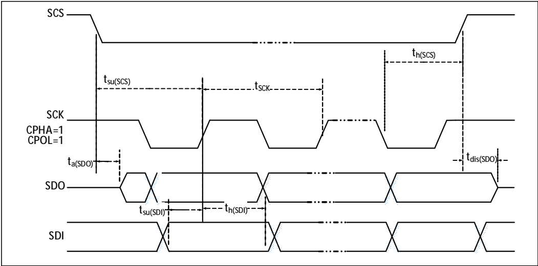
图 10-2 SPI 模式 3 时序图
