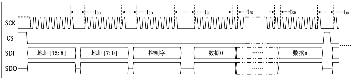
图 10-3 SPI 串行接口图
