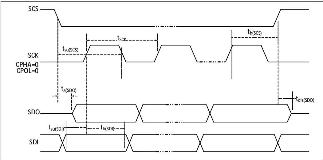
图 10-1 SPI 模式 0 时序图
