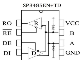
图 1 SP3485EN+TD引脚分布图
