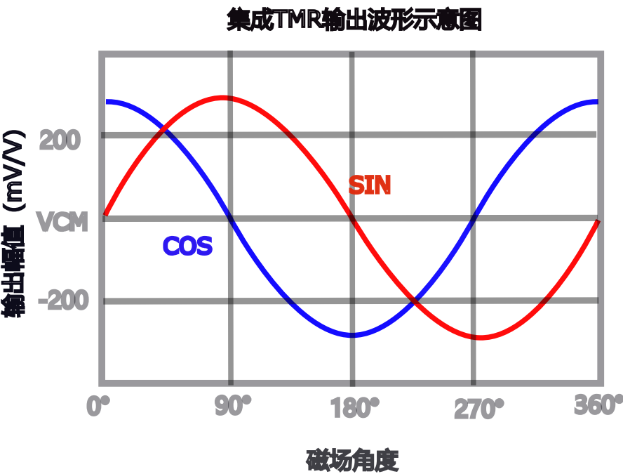
Figure 6: KTM5900 集成的 TMR 信号输出示意图
