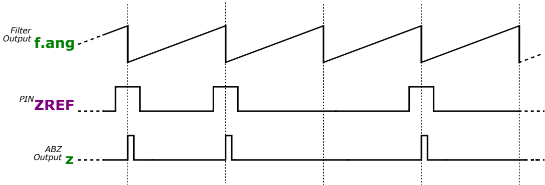
Figure 13: A.ZMOD = 10, 进行 Z 信号的选择示意图
