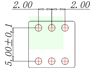
印制线路板 PCB Layout Recommended
