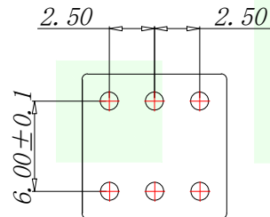
印制线路板 PCB Layout Recommended
