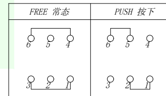
电路图 Circuit Diagram
