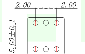
印制线路板 PCB Layout Recommended
